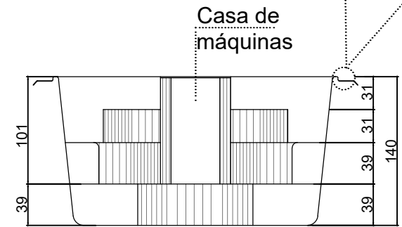
CORTE B Esc: 1:50
