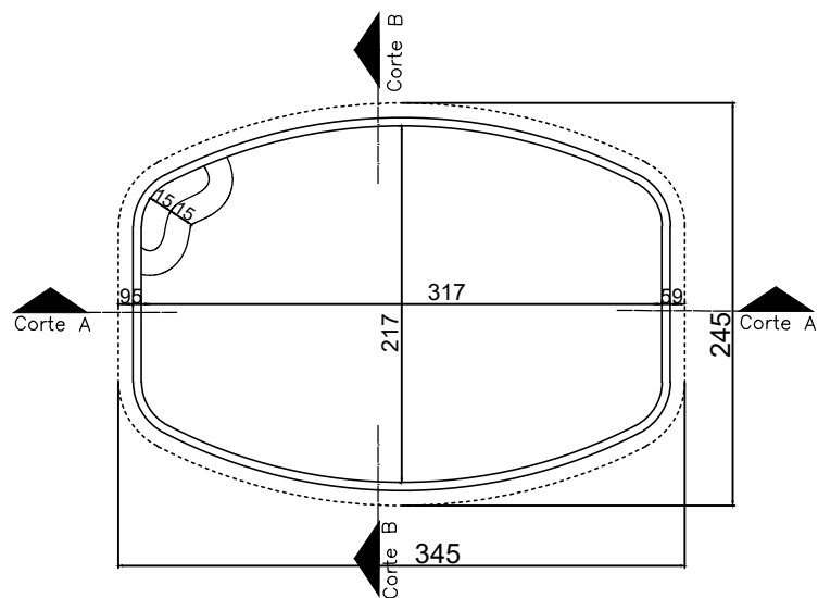
PLANTA BAIXA Esc:1:50
