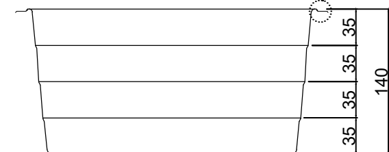
CORTE B
