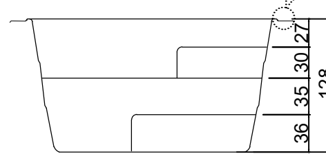
CORTE B Esc: 1:50
