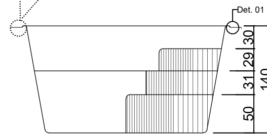
CORTE B Esc: 1:50
