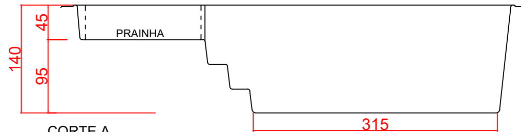
CORTE A
