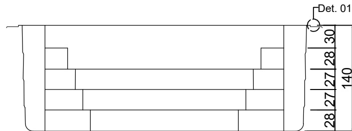
CORTE B
