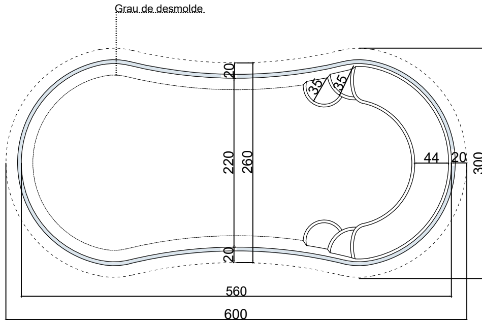
PLANTA BAIXA
