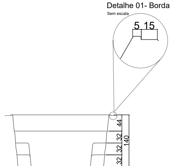
CORTE B
