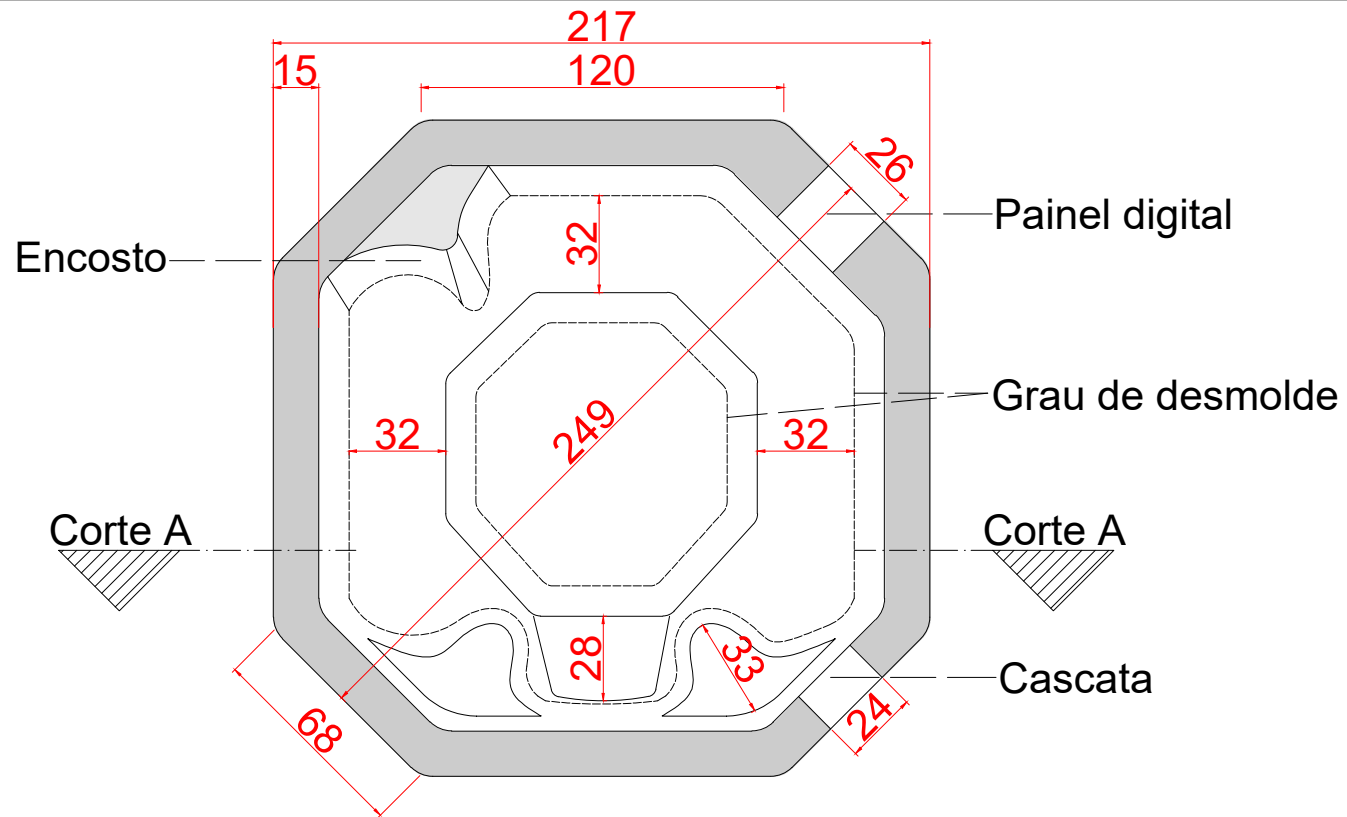
PLANTA BAIXA- MEDITERRANIC ESC:1/25
