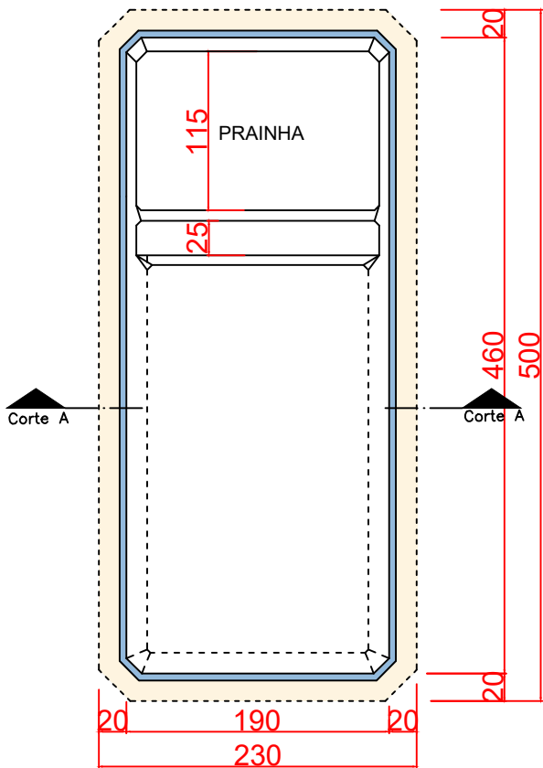
PLANTA BAIXA
